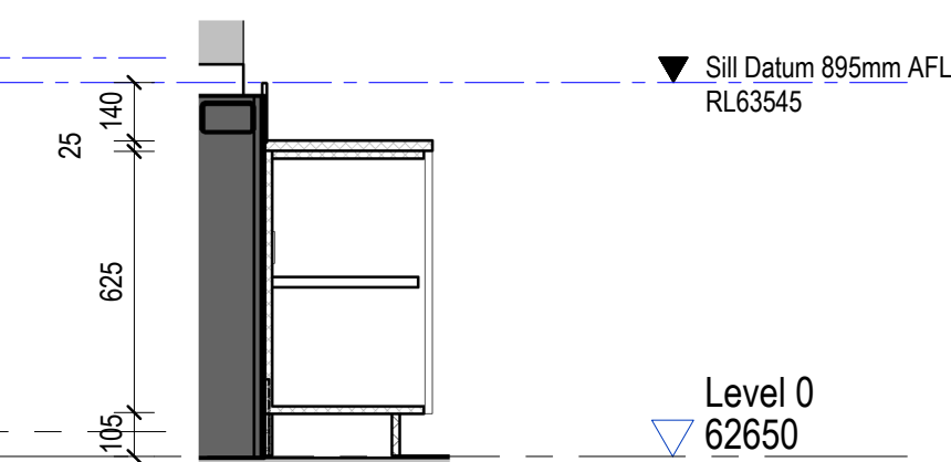
9 JO-BD-5b Section 1 : 20
