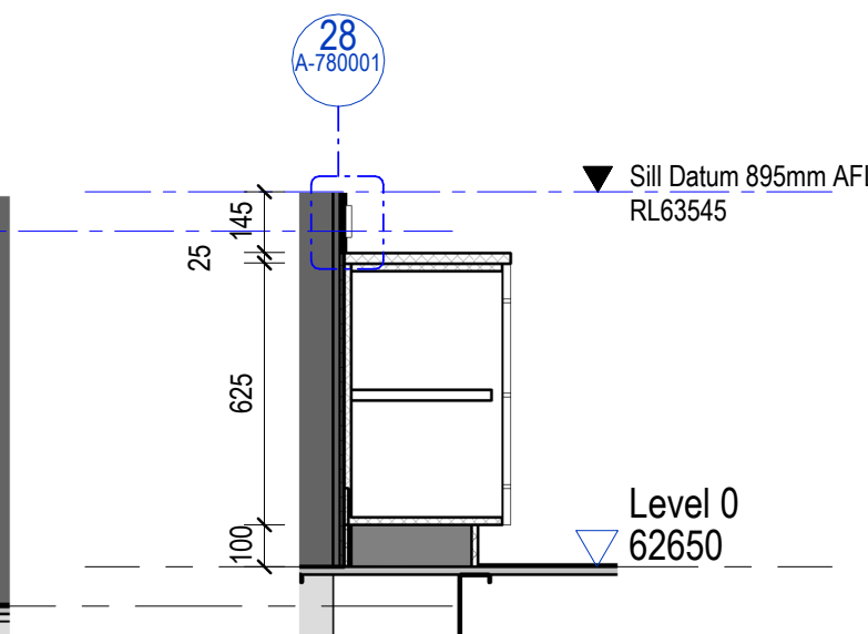
5 JO-BD-5a Section 1 : 20
