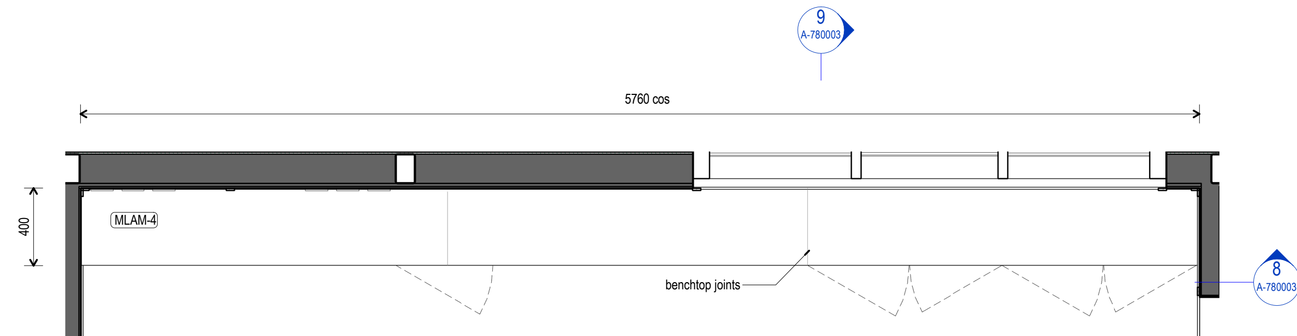
7 JO-BD-5b - Plan 1 : 20
